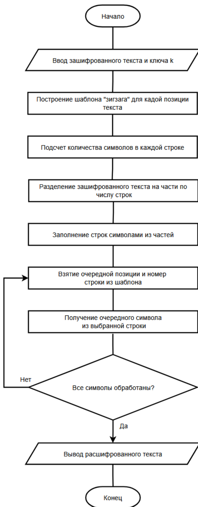
Рисунок 4.2 – Схема алгоритма дешифрования «штакетника»
