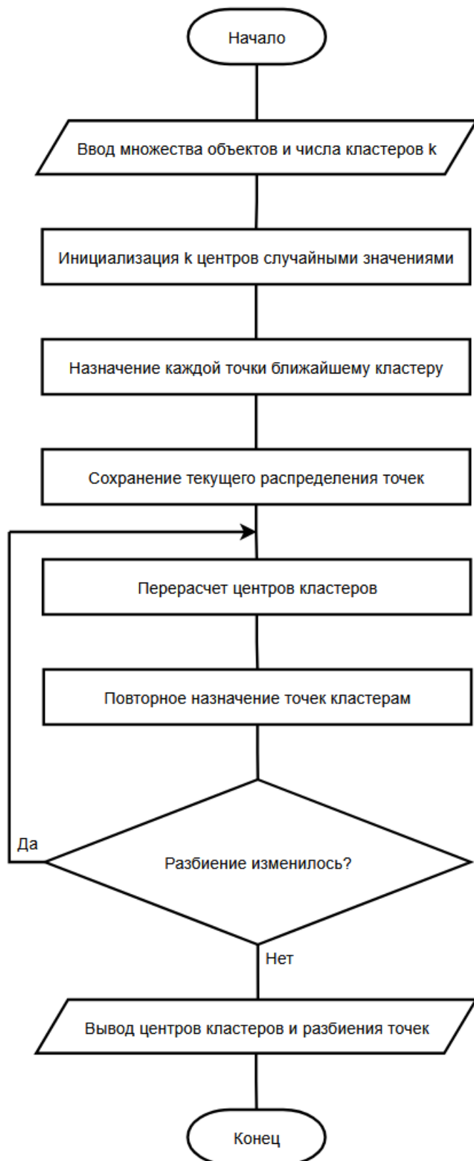
Рисунок 2.2 – Схема алгоритма k-means
